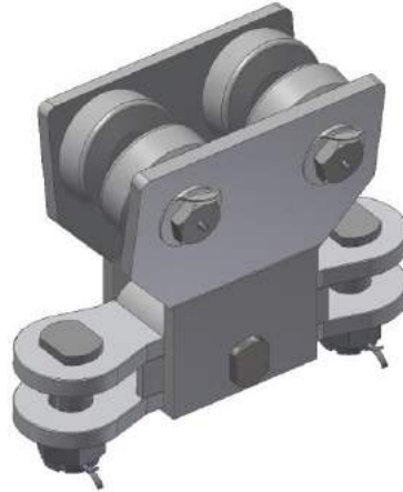
Рис. 2а – горизонтально-горизонтальное расположение сцепок.
