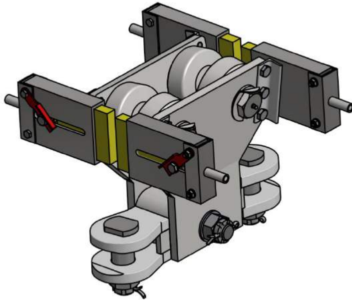
Рис. 4 – Тележка WTZB с двумя парами скребков.
