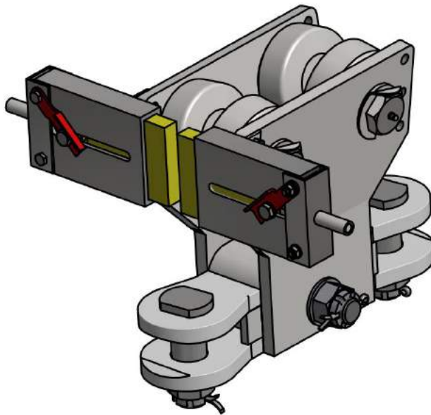
Рис. 5 – Тележка WTZB с одной парой скребков.
