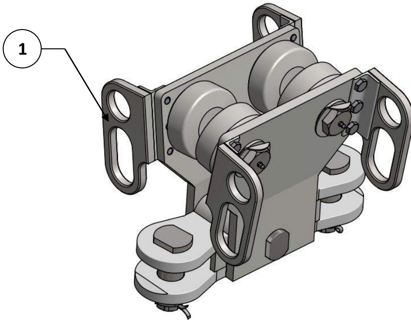
Рис.8 – тележка WTZB с 4 зажимами (1) для протягивания электрических кабелей, гидравлических шлангов и т. п.
