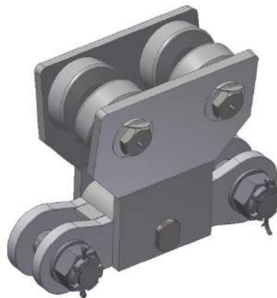
Рис. 2б – горизонтально-вертикальное расположение сцепок.
